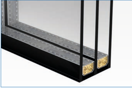
Treglaspaket 4x18x4x18x4 VÄRME OCH LJUSINSLÄPP
