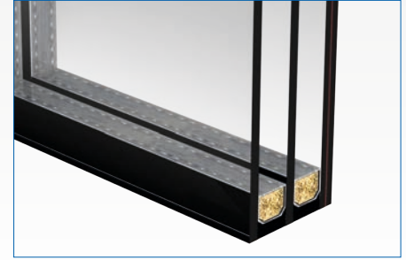
Treglaspaket 4/14/4/14/33.1 VÄRME OCH SÄKERHET
